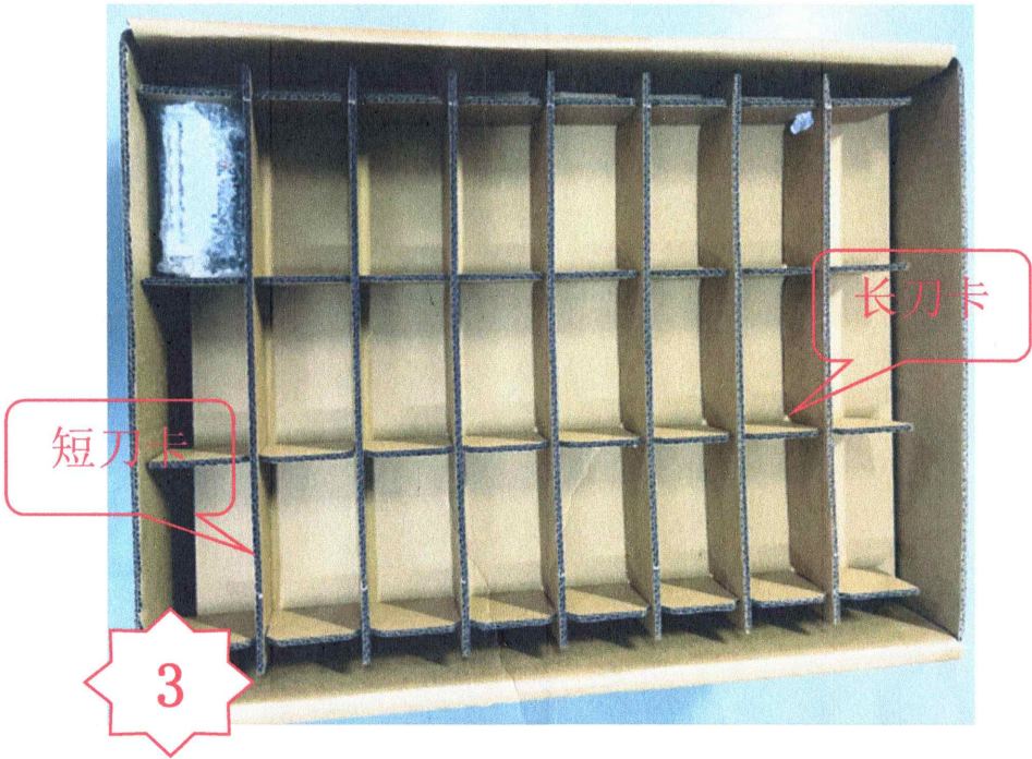
图三, 将 PA1038 如图装入内箱内, 每层 24PCS, 每箱 3 层的方式包装, 同时在底部和每层顶部各放一块隔板, 共 4 块隔板。
