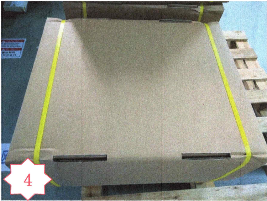
图四, 确认 PA1038 无漏装后, 将 22 的内箱与外箱配合并打包装带待出货。
